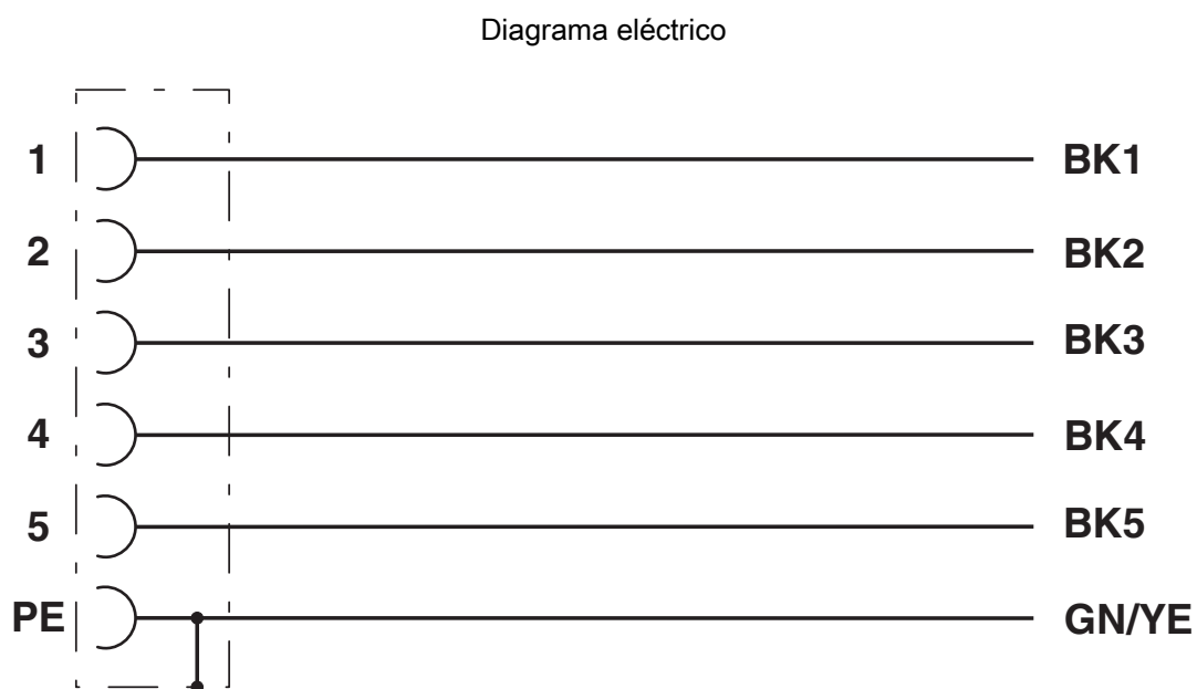
Ocupación de contactos del conector hembra M12
