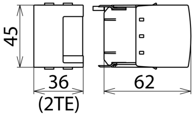
Dimensioni DGP M MOD 255
