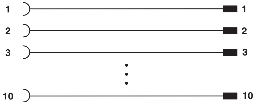
Schaltplan
