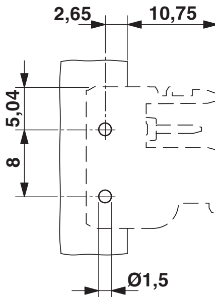
Gabarit perçage / géom. pastille soudage
