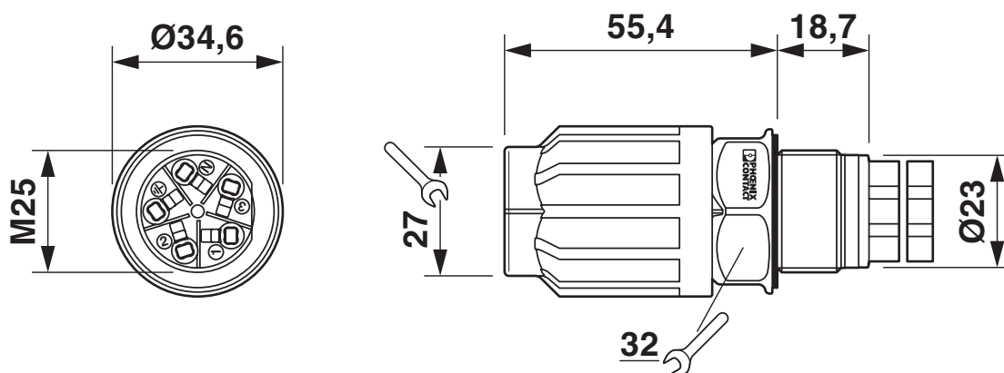
Esquema de dimensiones: QPD W...
