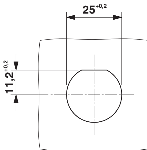
Dessin coté
