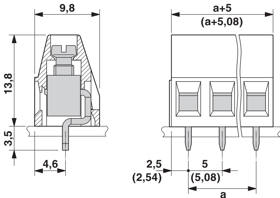
Dessin coté
