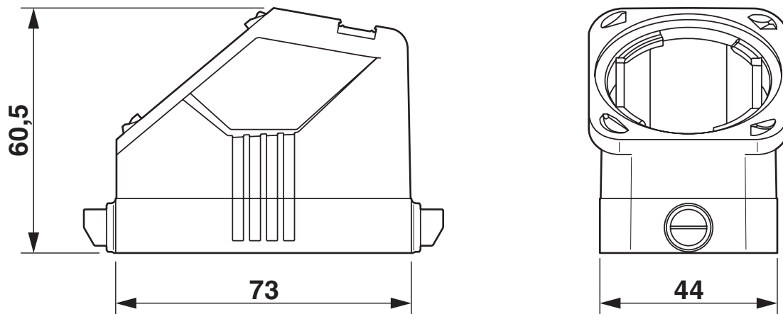
Maßzeichnung
