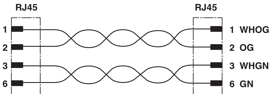
Schaltplan
