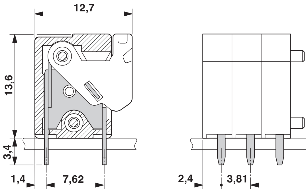
Maßzeichnung
