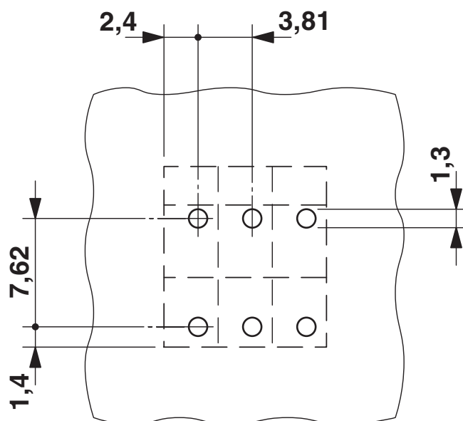
Bohrplan/Lötpadgeometrie
