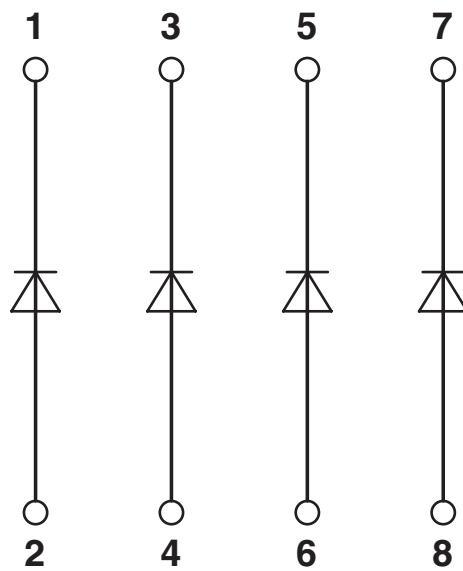
Diagrama eléctrico
