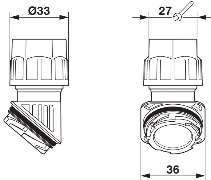
Maßzeichnung
