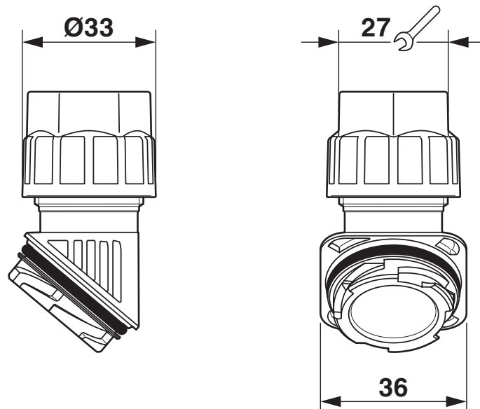
Dessin coté
