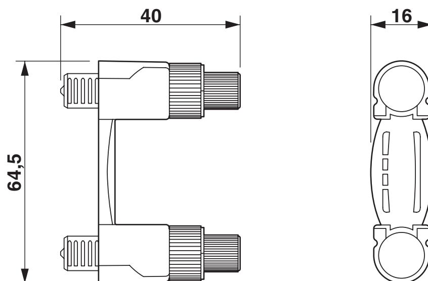
Dessin coté
