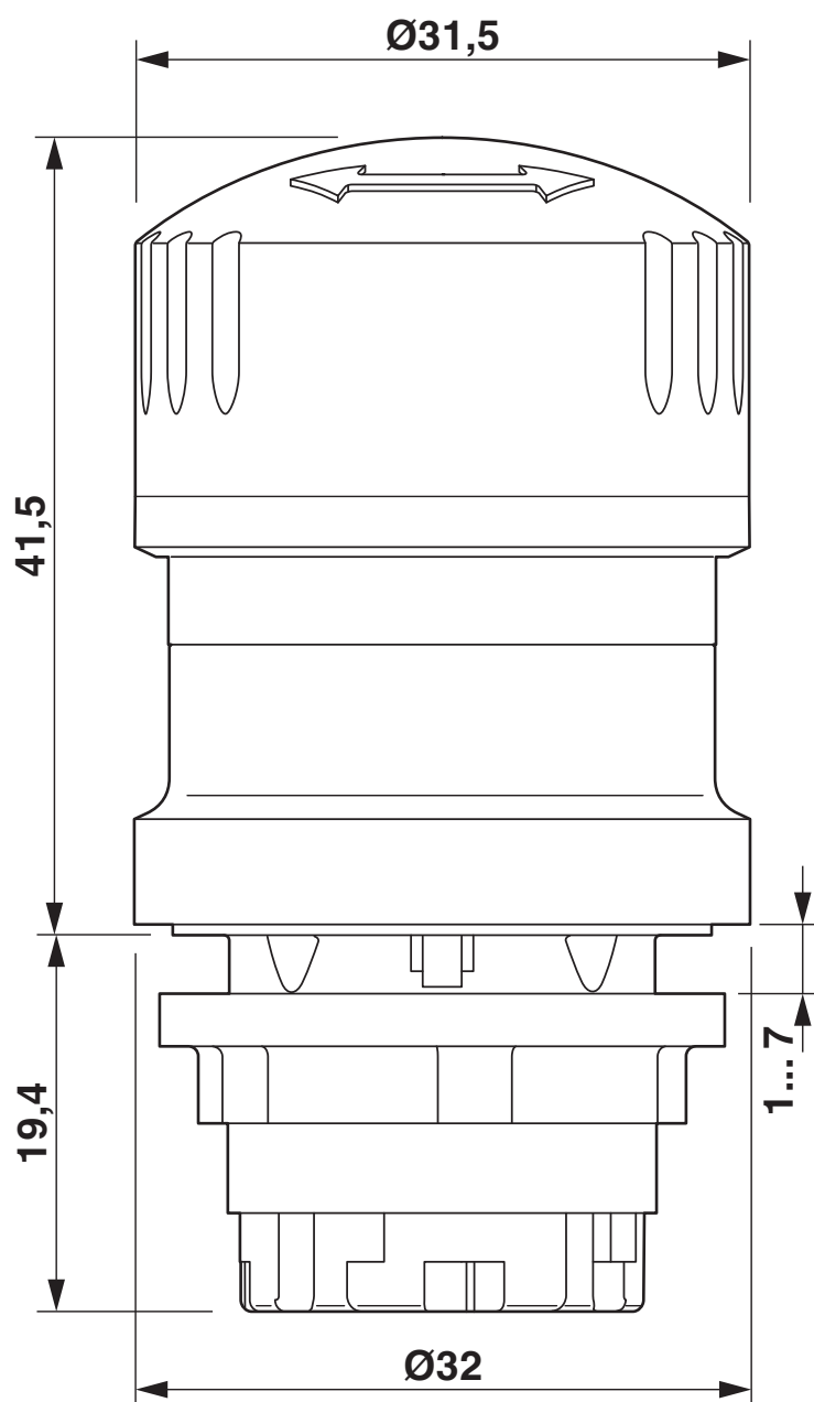
Dessin coté
