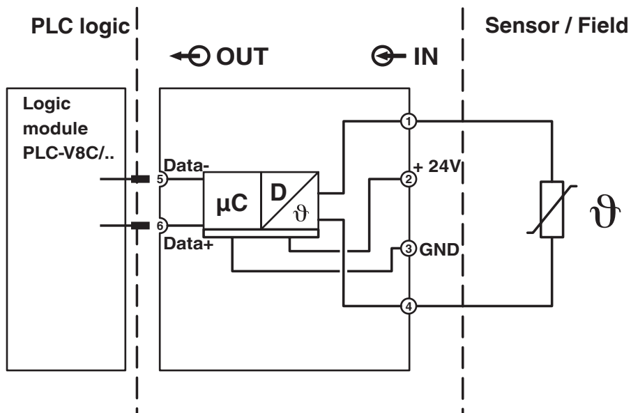
Schéma fonctionnel
