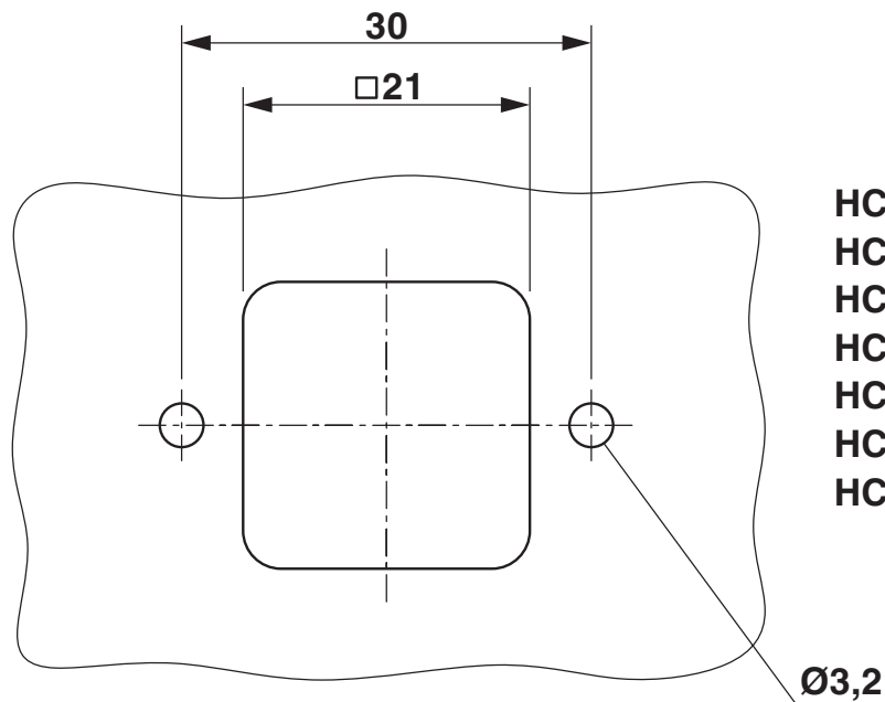
Dessin coté
