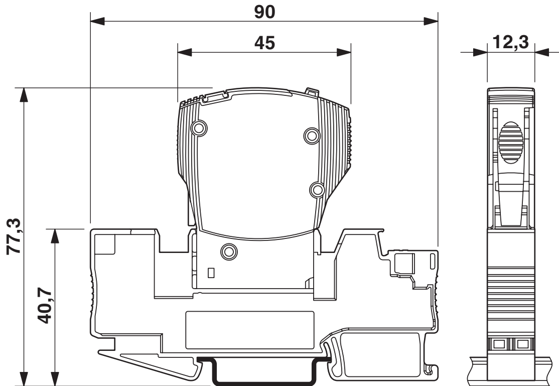
Dessin coté
