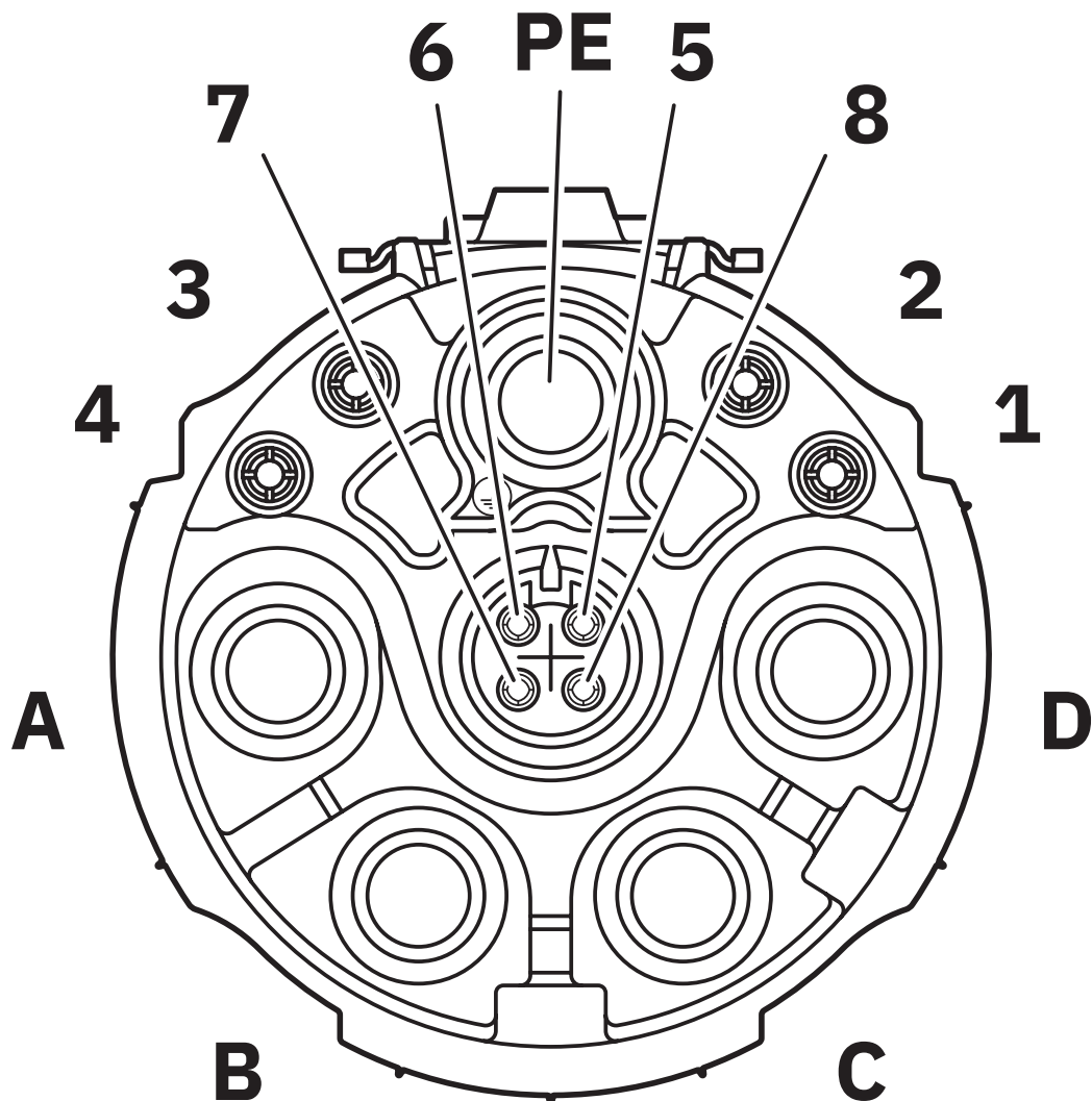
Esquema de polos conector hembra señal, codificación 1
