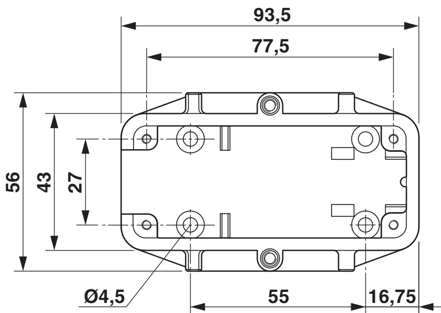
Esquema dimensiones vista desde arriba
