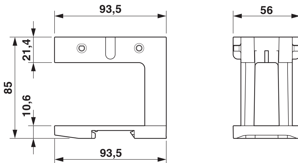
Dessin coté
