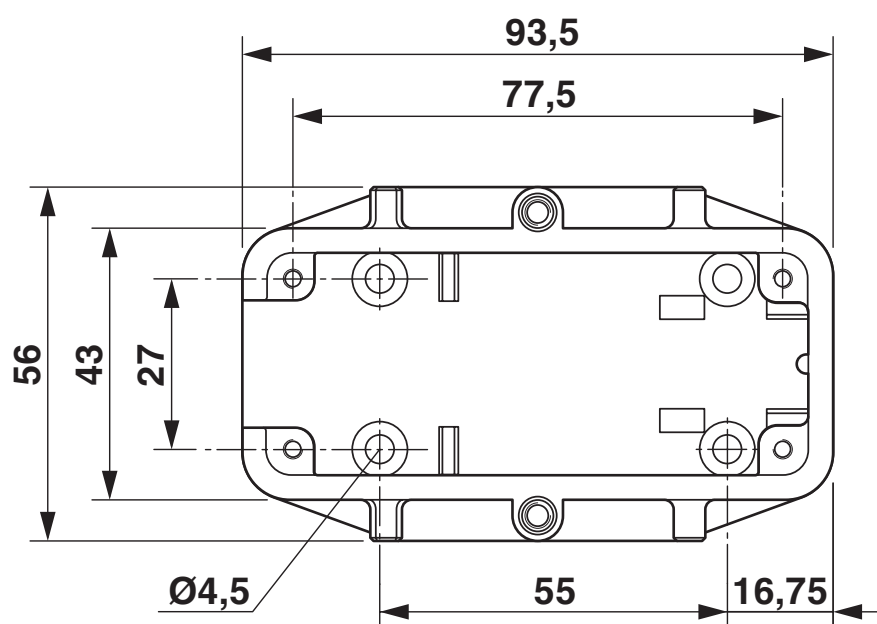
Dessin coté
