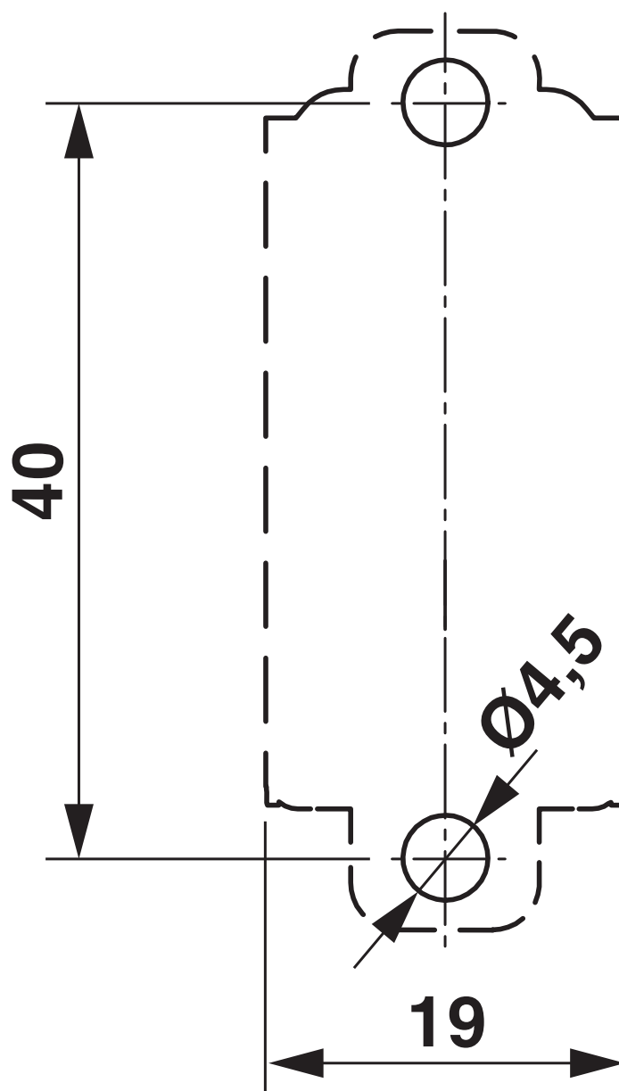
Esquema de taladros/geometría pads soldadura
