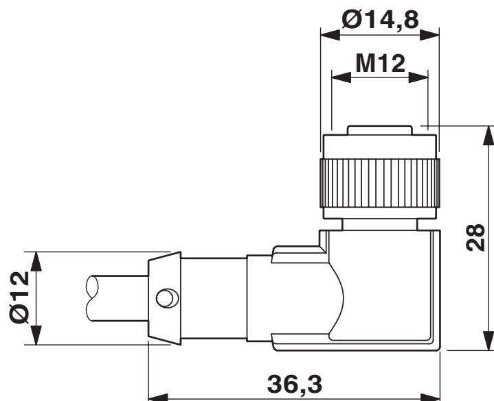
Maßzeichnung
