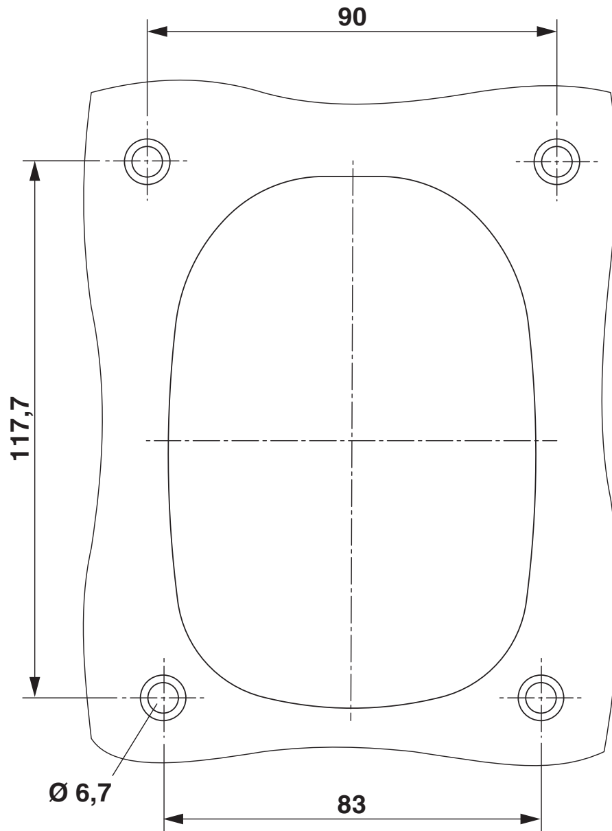
Bohrplan/Lötpadgeometrie
