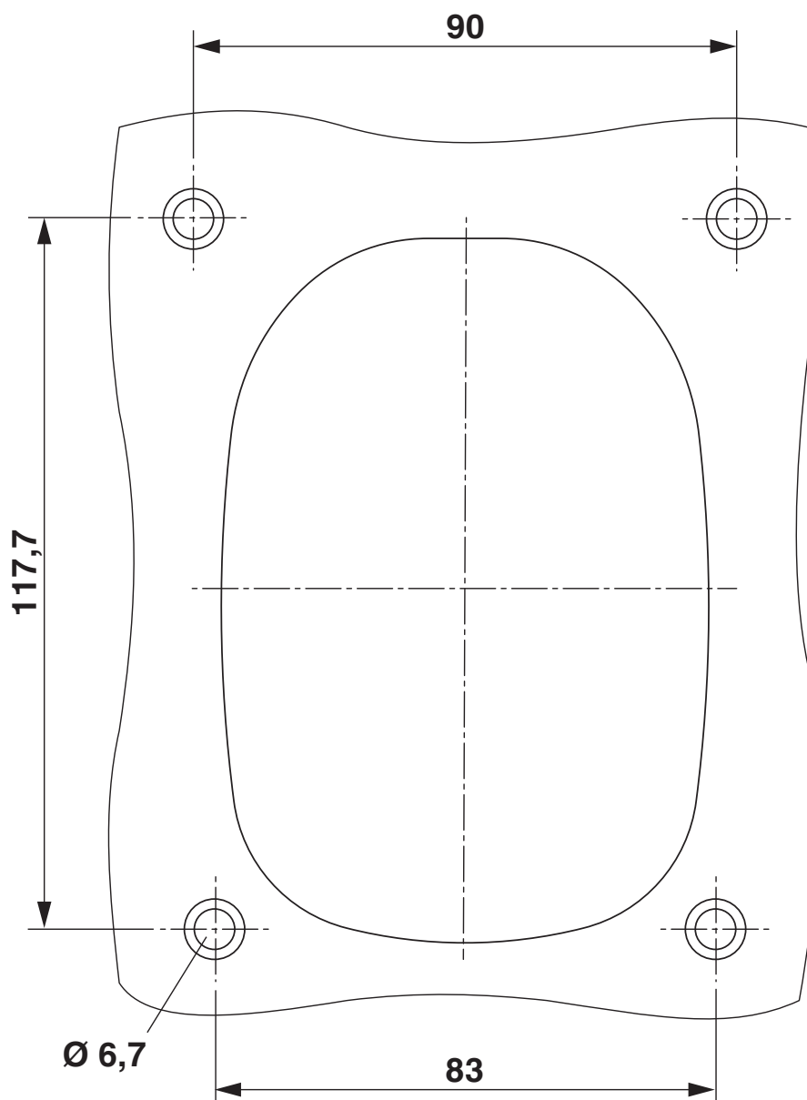
Esquema de taladros/geometría pads soldadura
