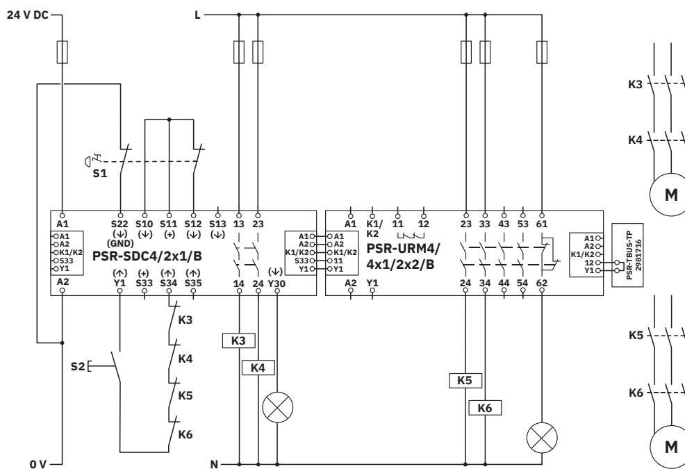
Zweikanalige Not-Halt-Überwachung mit Kontakterweiterung
