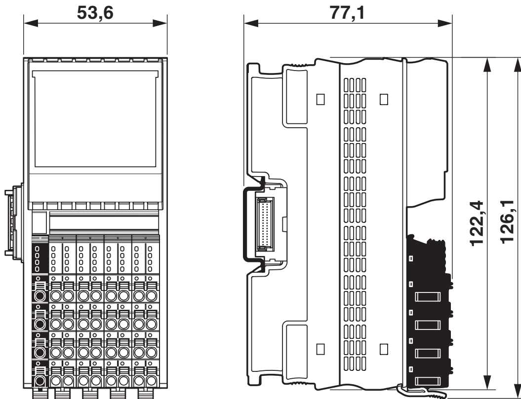
Maßzeichnung
