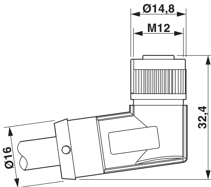
Conector hembra SPEEDCON M12, acodado, apantallado
