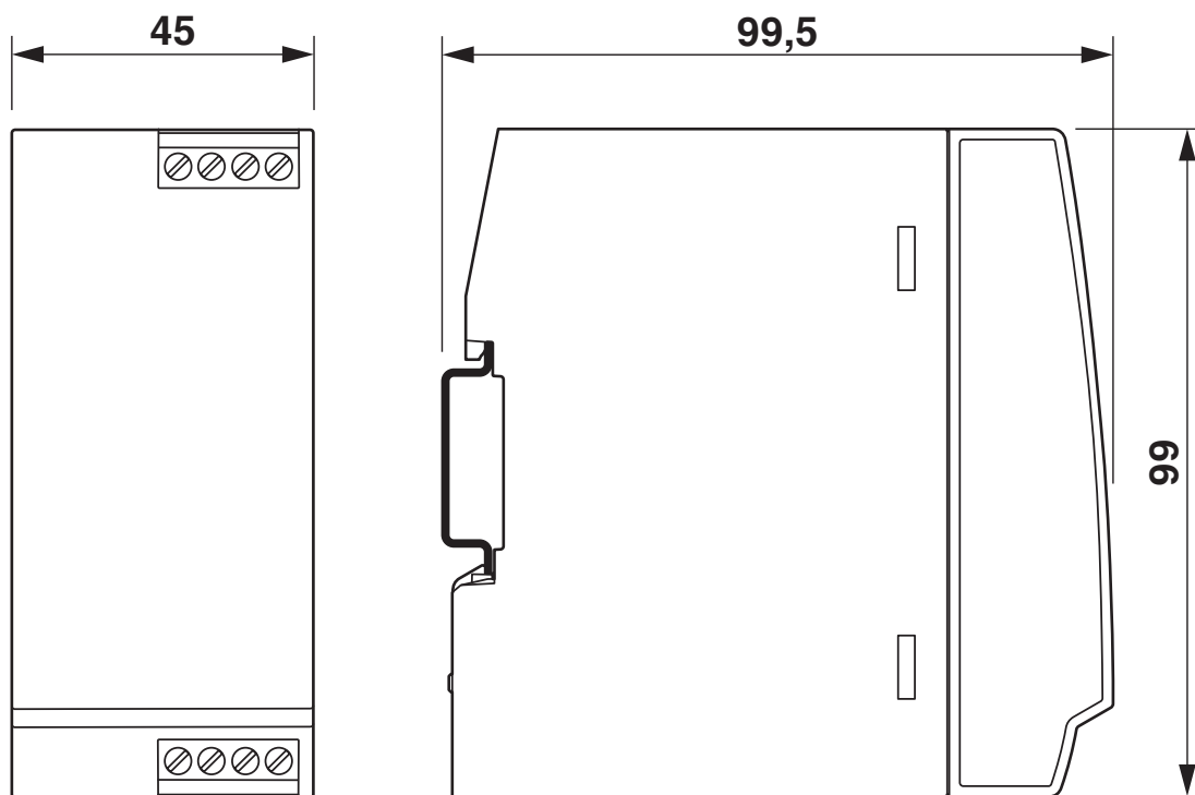
Dessin coté
