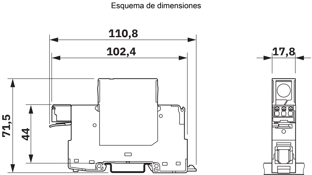
Plano esquemático
