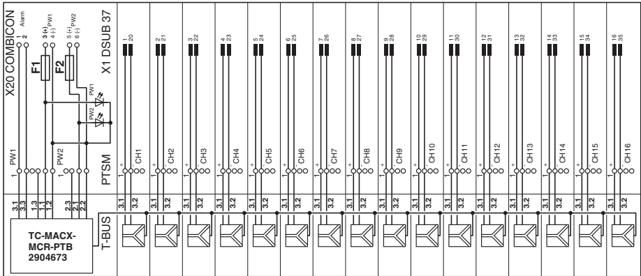
Diagrama eléctrico
