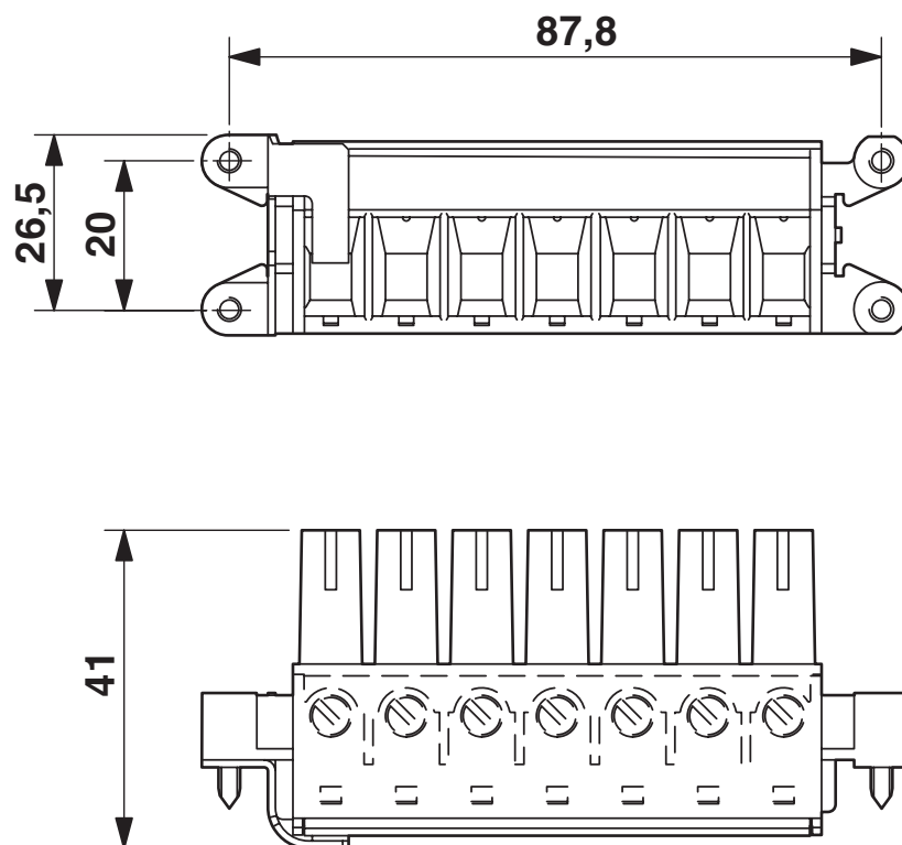
Dessin coté
