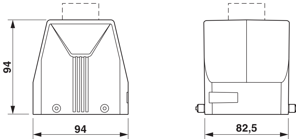
Maßzeichnung
