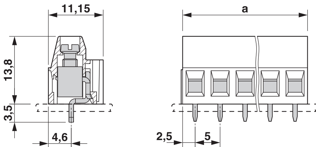
Dessin coté
