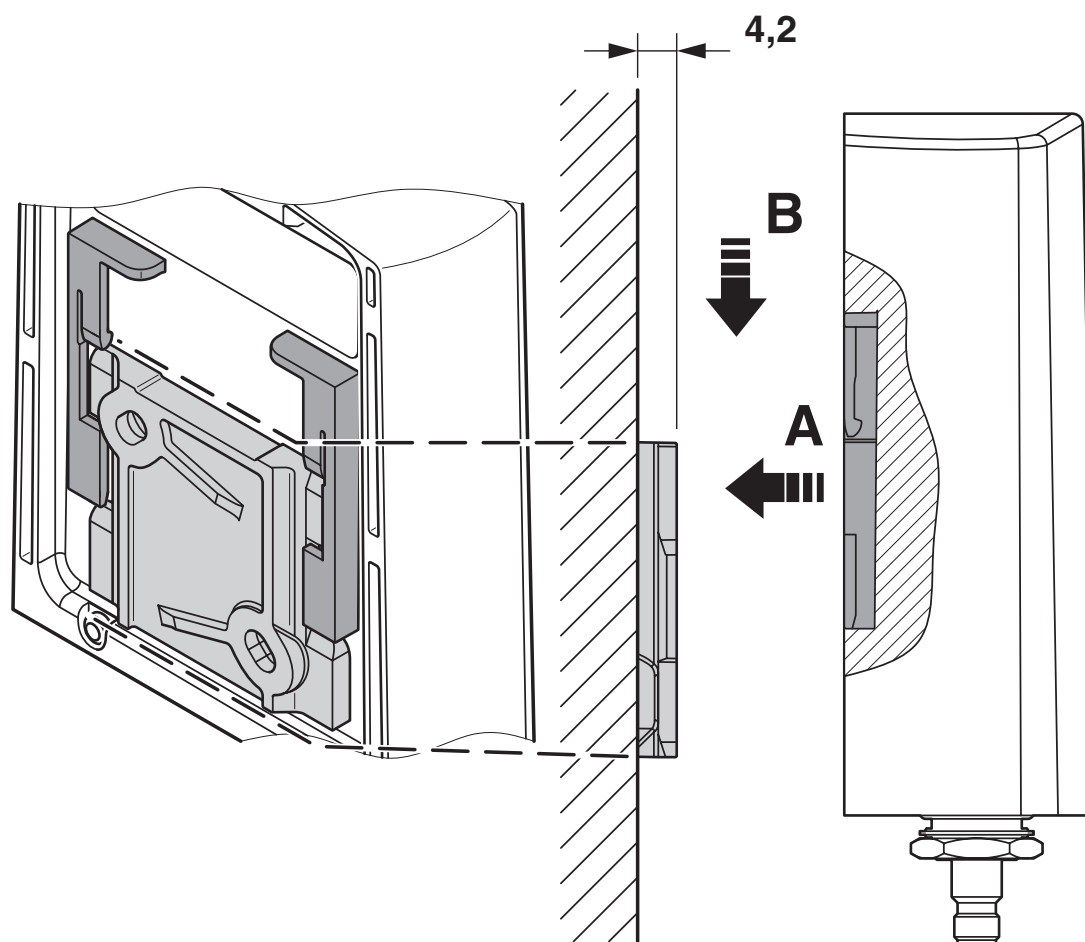
Dessin schématique
