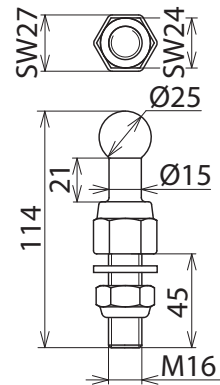
Maßbild KFP 25 M16 45 SKM
