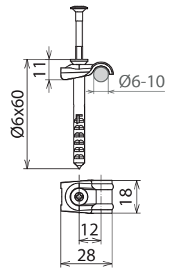
Maßbild LH DQ 6.10 ND6X60 V2A
