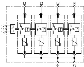
Esquema del DG M TNS 275 FM
