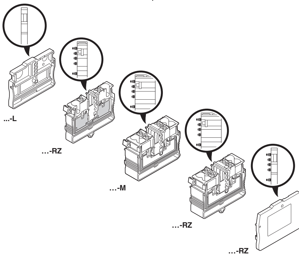
Plano esquemático
