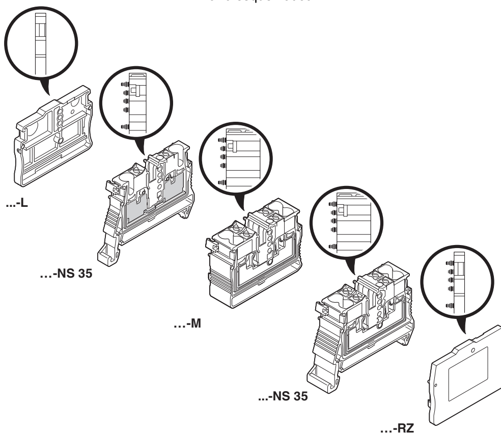
Plano esquemático
