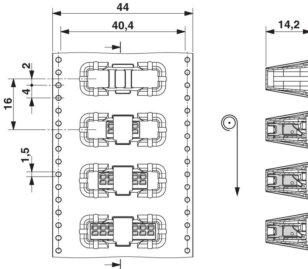
Dessin coté
