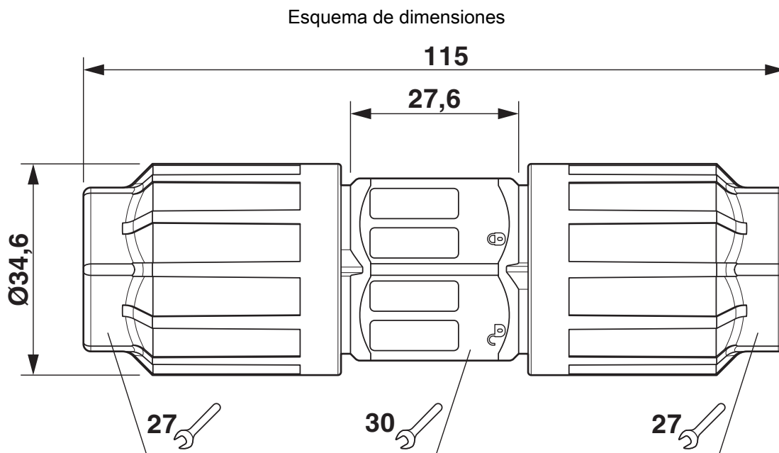
Dibujo acotado QPD C 5 x 2,5
