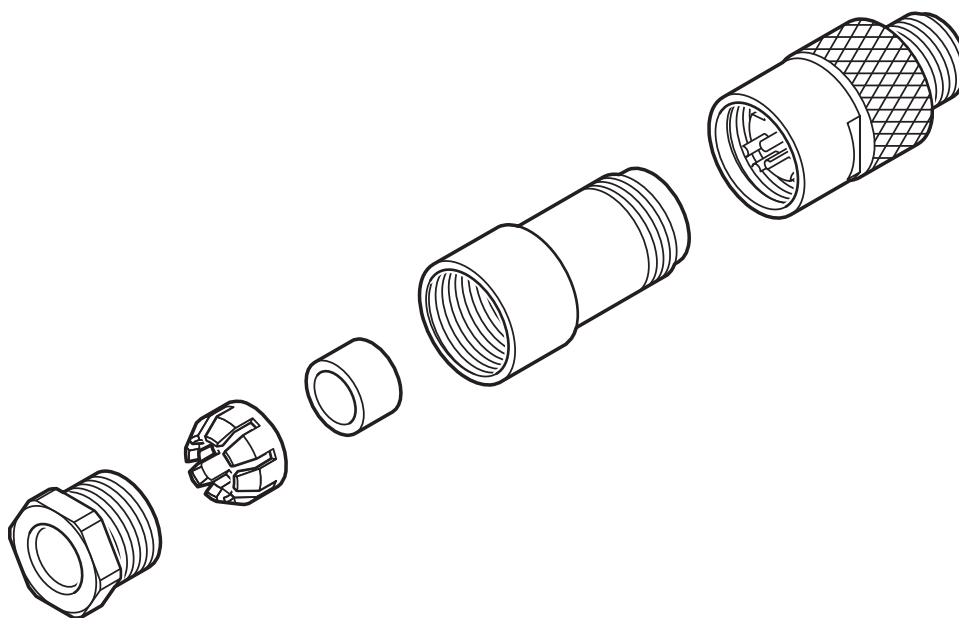
Plano esquemático
