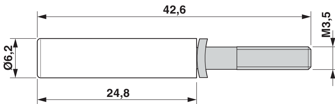
Dessin coté
