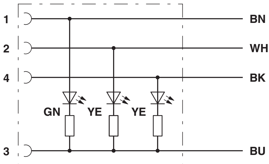
Ocupación de contactos de las hembras M12 con LED
