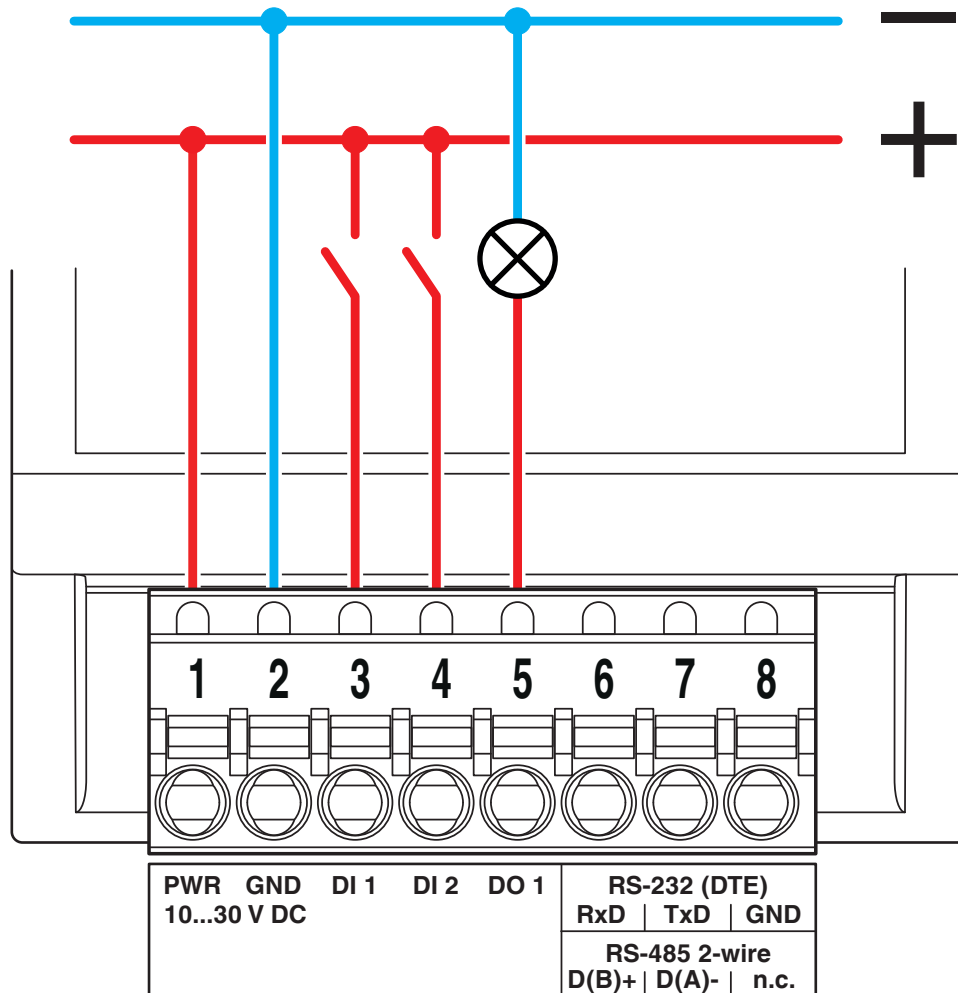
Anschlusszeichnung
