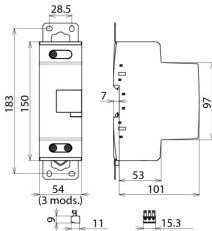
Dimensioni DBM 1 CI 440 FM
