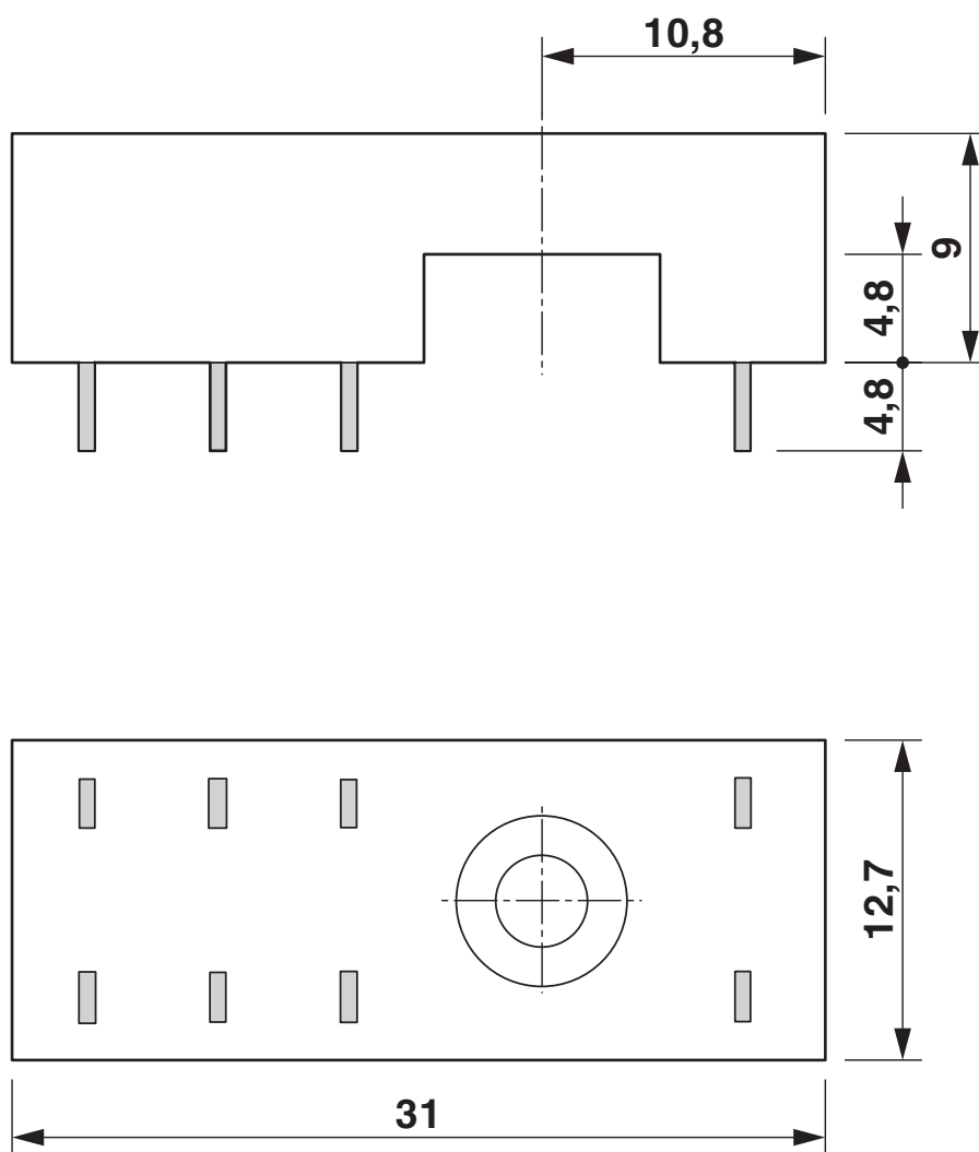
Dessin coté
