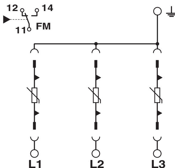
Diagrama eléctrico
