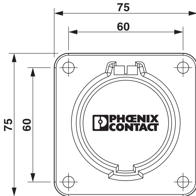
Maßzeichnung
