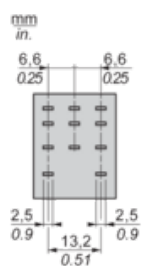
Stecker-Seitenansicht
